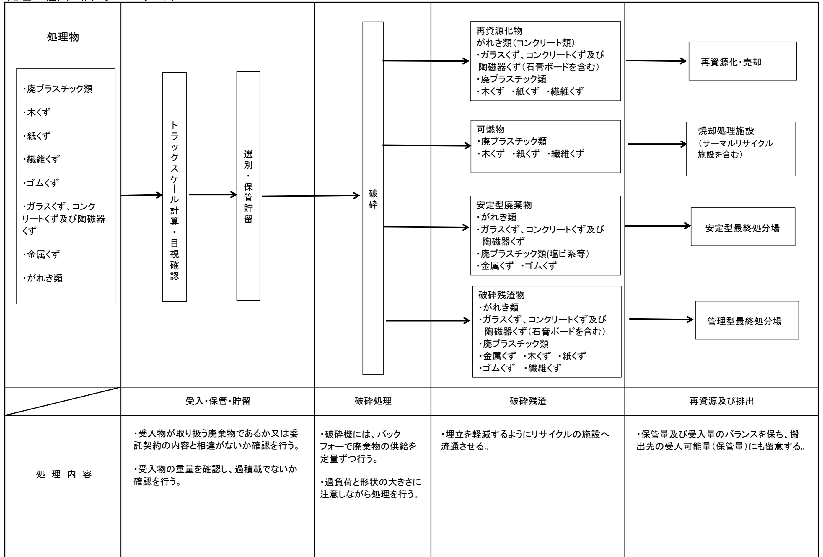
処理工程図（姉崎エコプラント）
